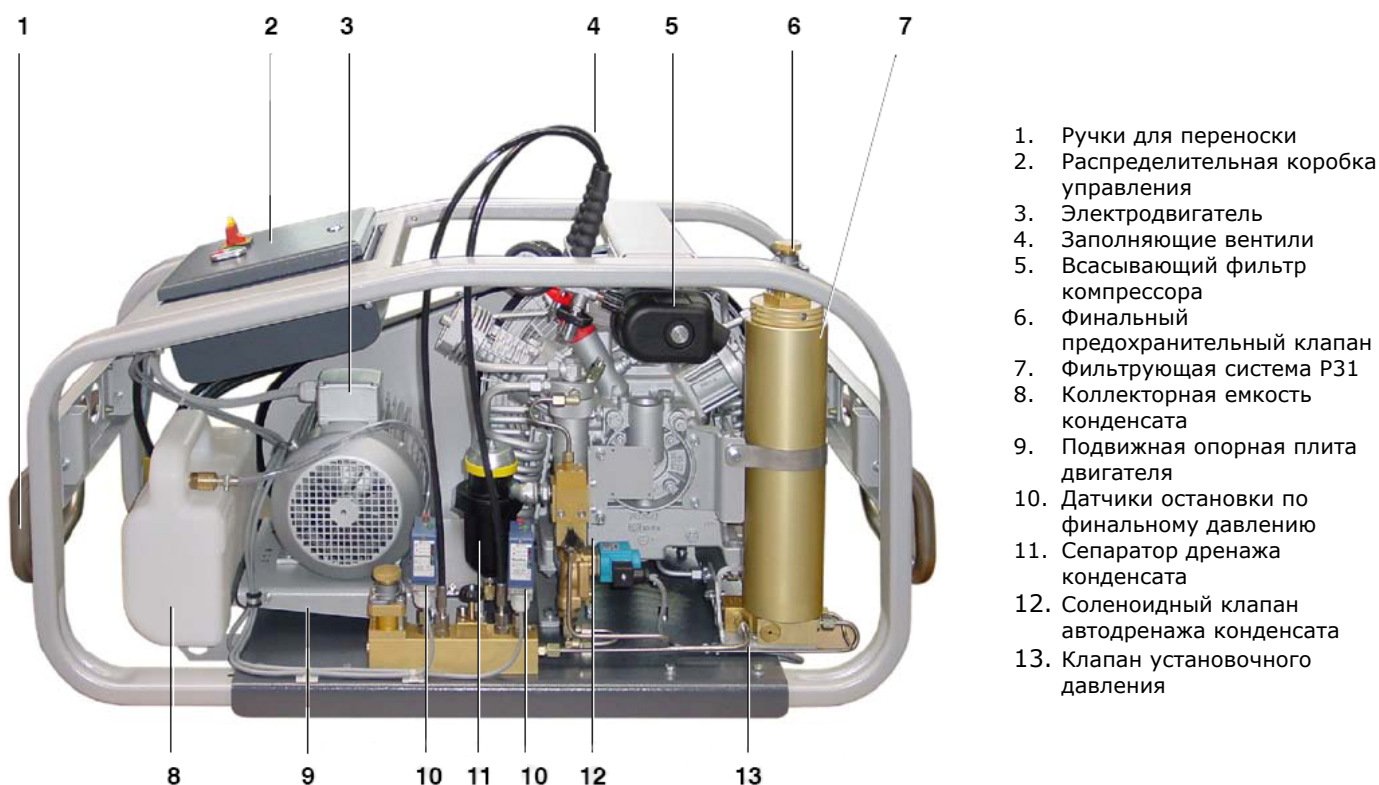
Рис.2. Компрессор Mariner 200 с электроприводом, фильтрующей системой P31, переключателем на два давления и автоматикой сброса конденсата
