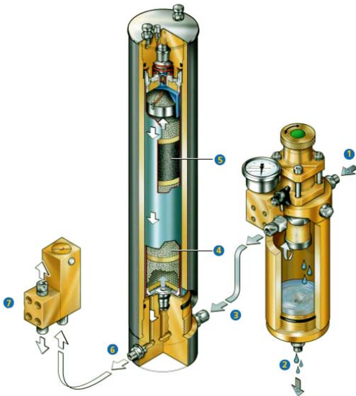
Рис.28. Фильтрующая система P41
