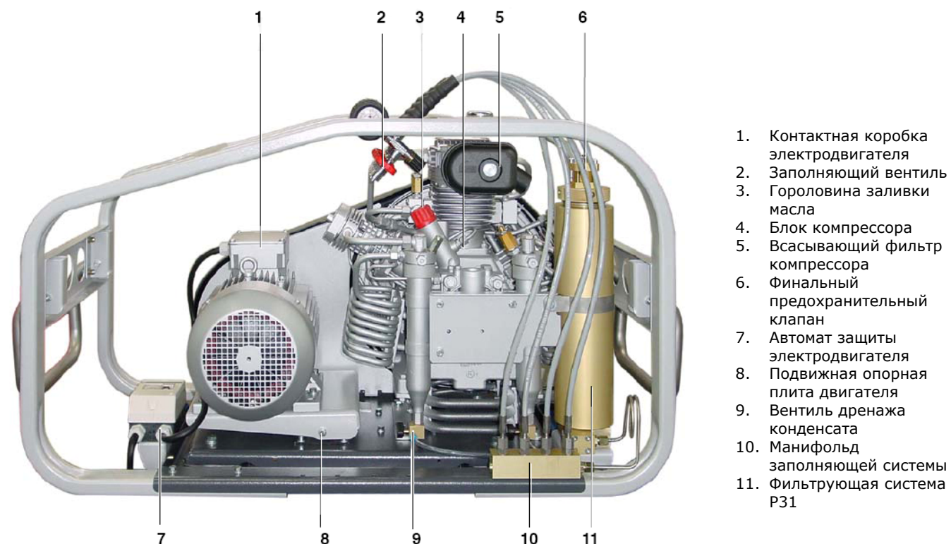
Рис.4. Mariner 200 с электроприводом в стандартной комплектации с двумя дополнительными шлангами
