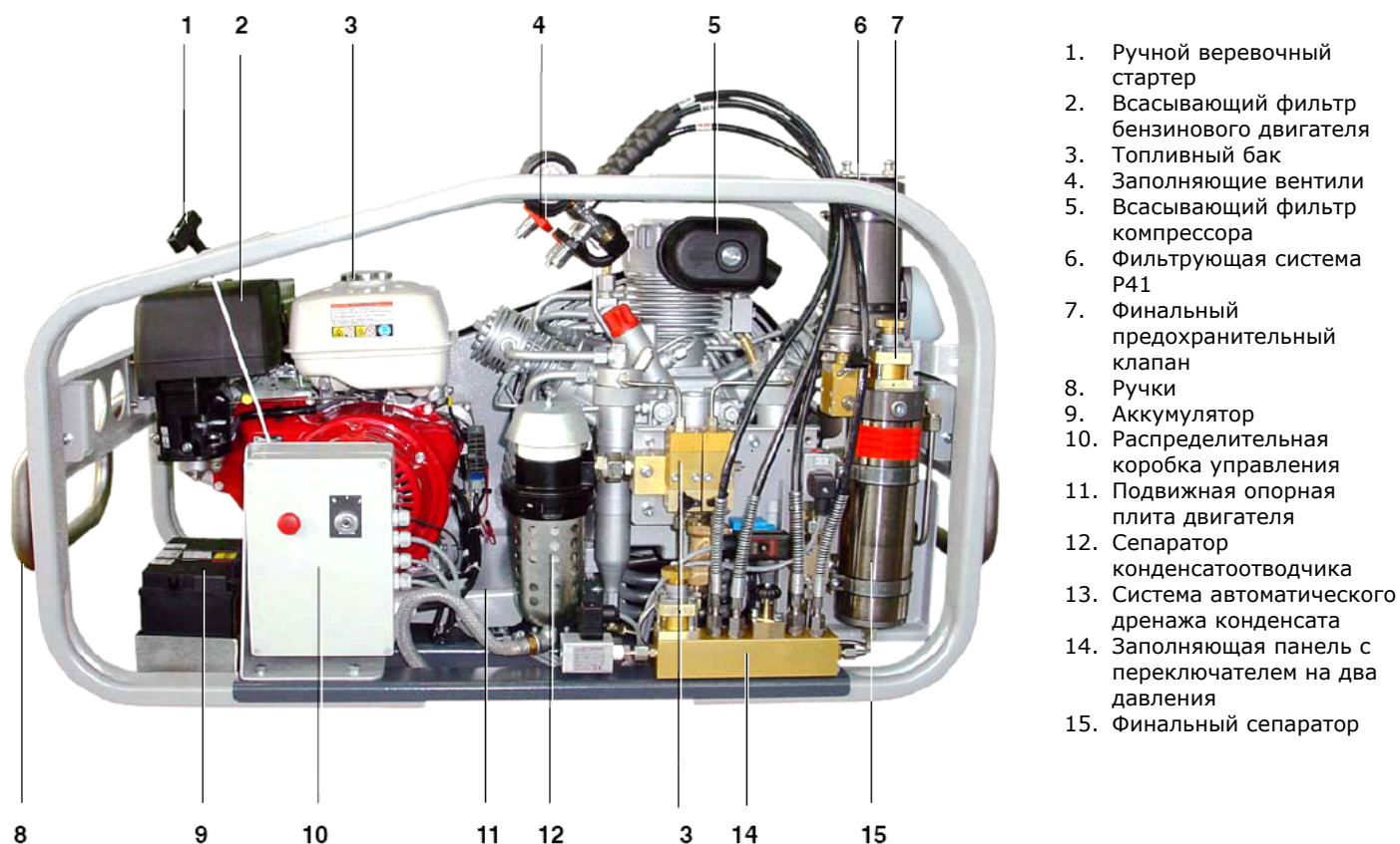
Рис.5. Mariner 200 с бензиновым двигателем, автоматикой сброса конденсата, автостопом по финальному давлению и фильтрующей системой P41
