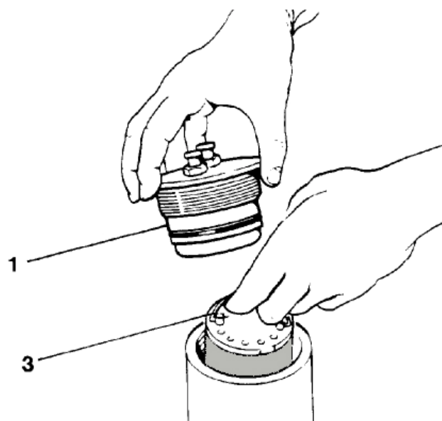
Рис.31. Замена картриджа
