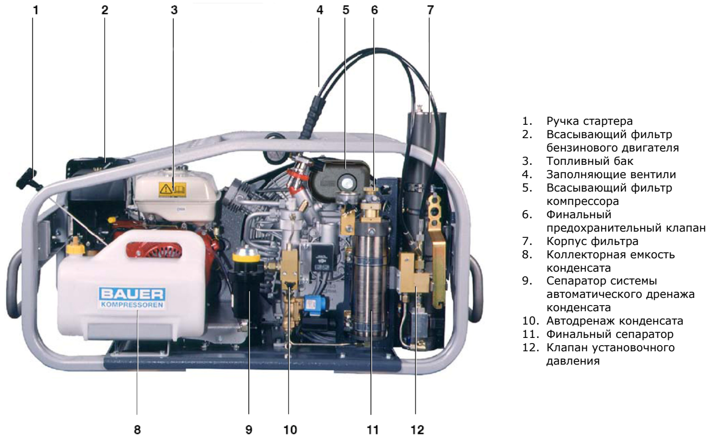
Рис.3. Компрессор Mariner 200 с бензиновым приводом, фильтрующей системой P41 и автоматикой сброса конденсата
